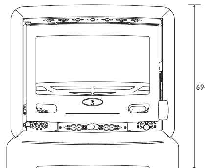
WIDOK Z PRZODU Z ZAMONTOWANĄ ŻELIWNĄ RAMĄ (6" RURA PRZYŁĄCZENIOWA)
